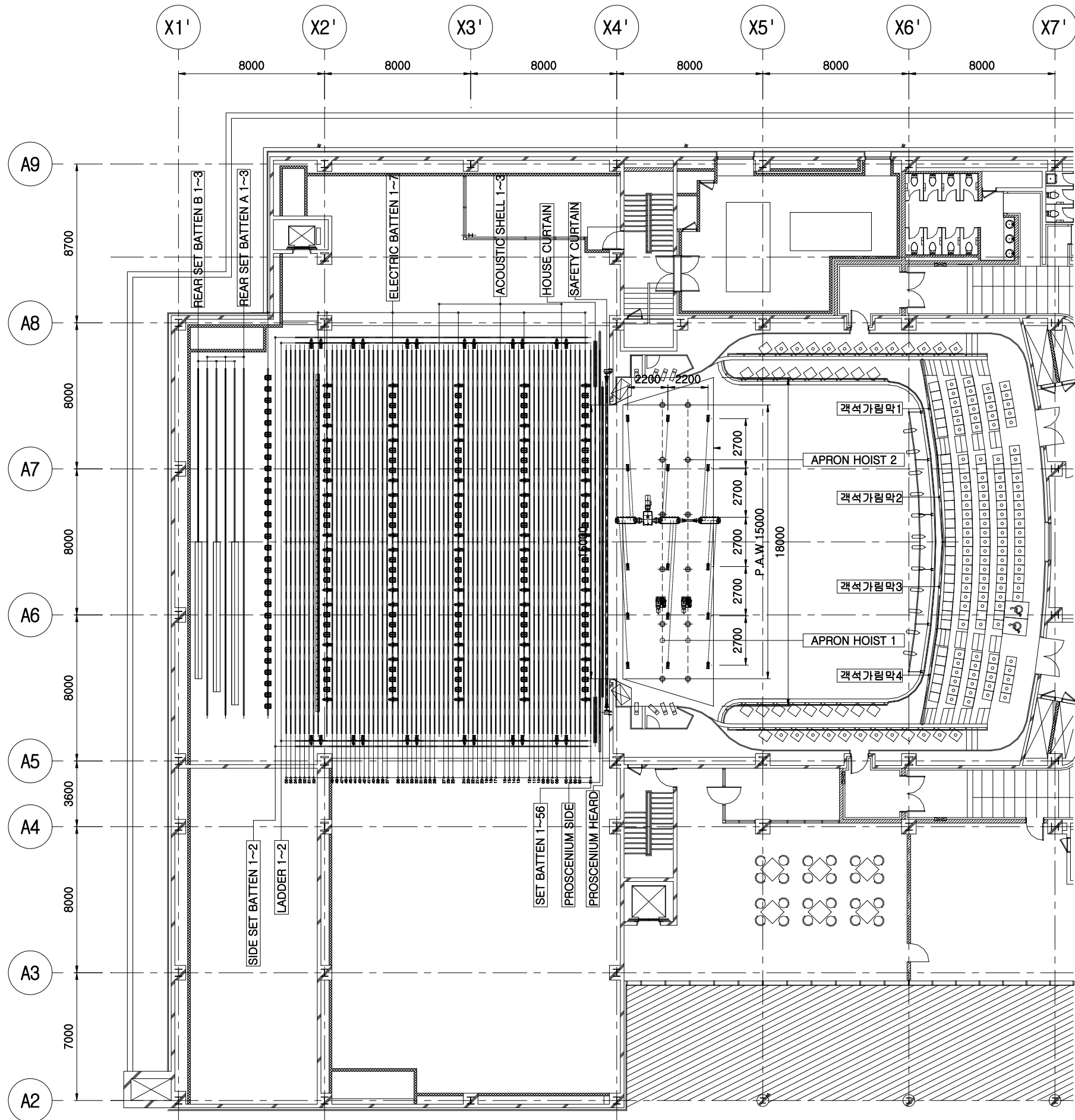
1 상부무대기계장치 평면도 KD103
