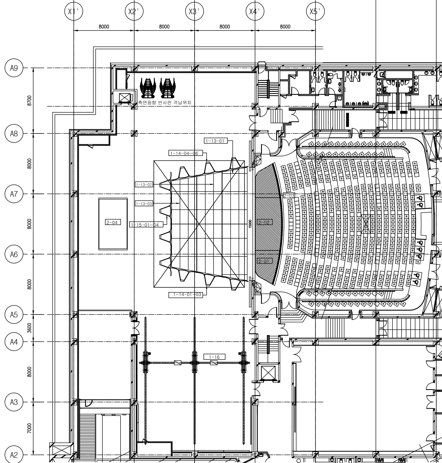
하부무대기계장치 평면도 KD104
