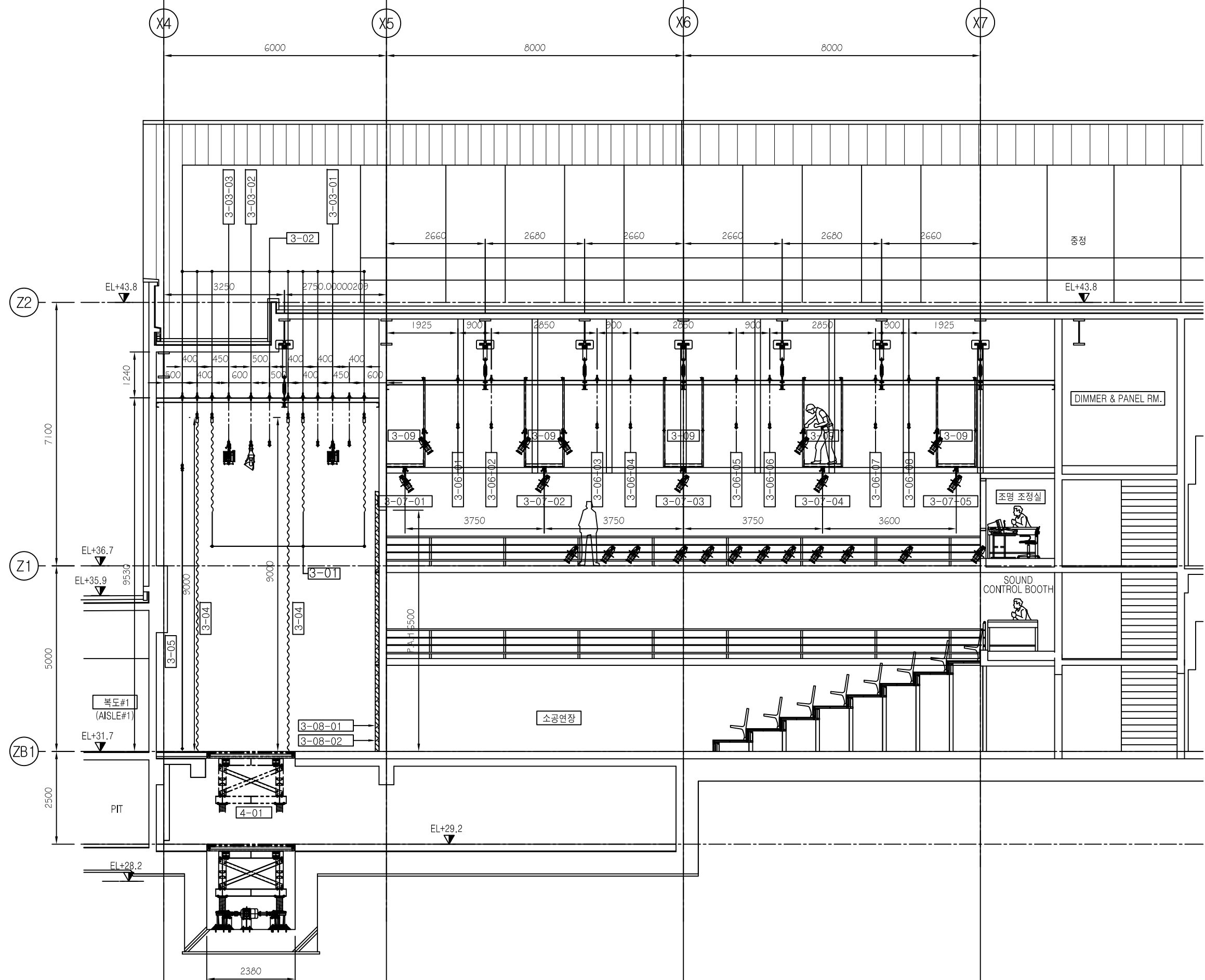
극장 드림 단면도
